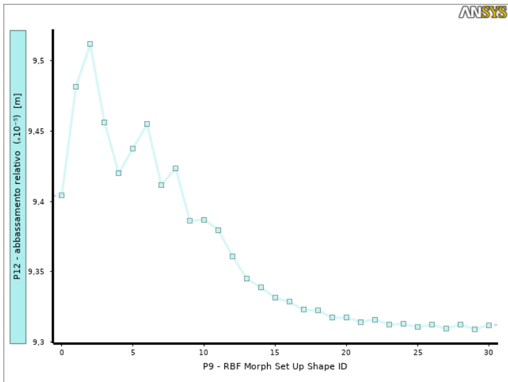
Figura 8: Abbassamento relativo tra le sezioni estremali della semi-spira
