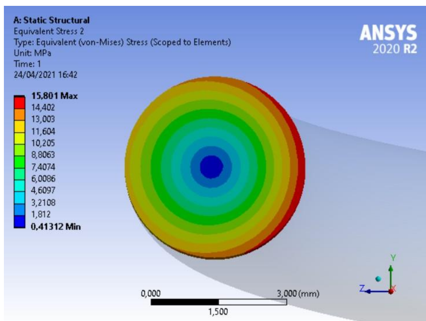
Figura 4.10: Tensioni di Von Mises sulla generica sezione del filo d'elica originario
