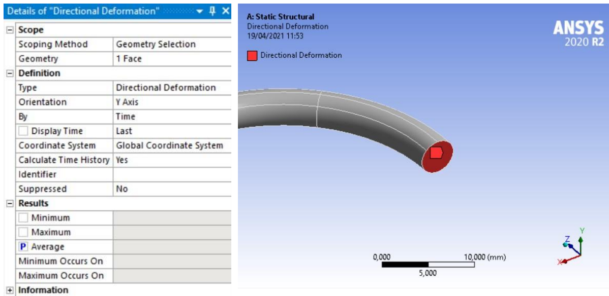
Figura 3.17: Abbassamento della sezione parallelo all'asse della semi-spira
