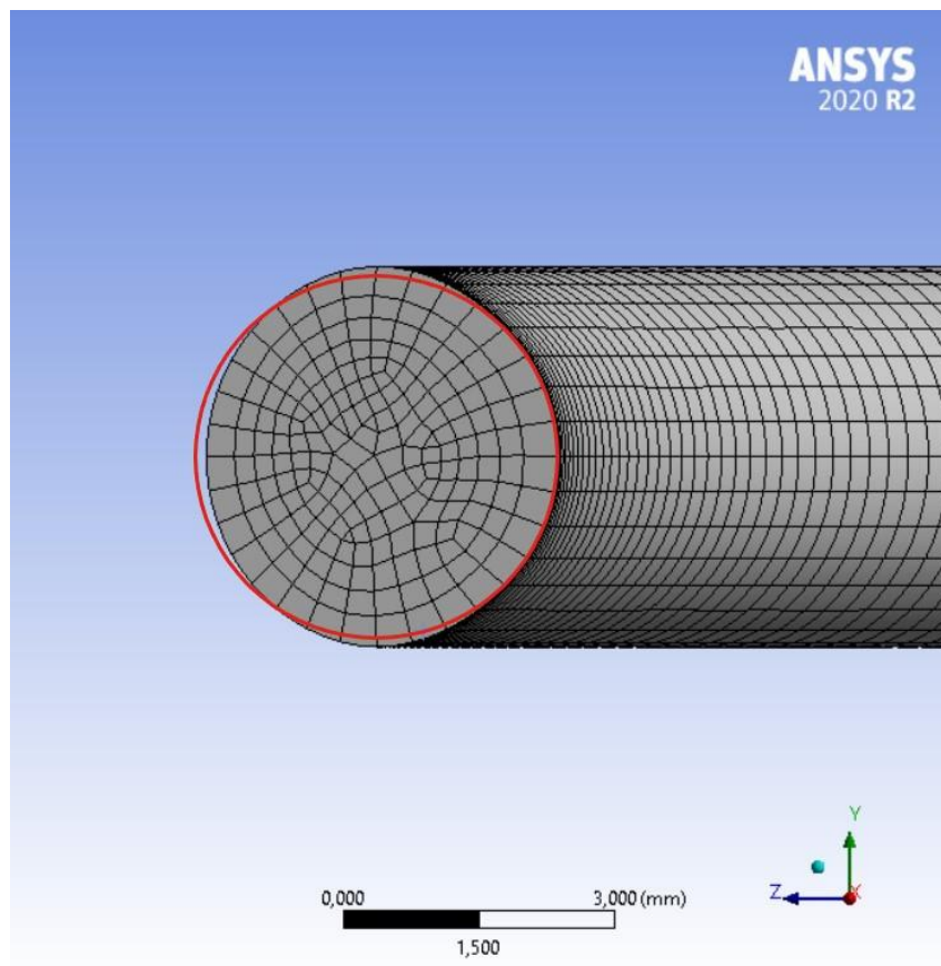
Figura 4.6: Sezione della semi-spira finale confrontata a quella originaria
