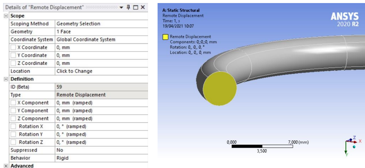
Figura 3.10: Settaggio dell'oggetto Remote displacement
