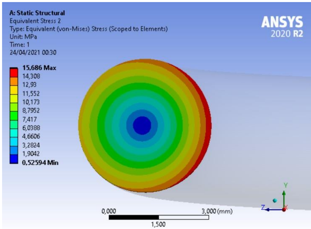
Figura 4.4: Tensioni di Von Mises sulla generica sezione della semi-spira originaria
