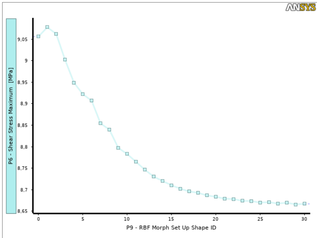
Figura 5: Sforzi tangenziali all'intradosso
