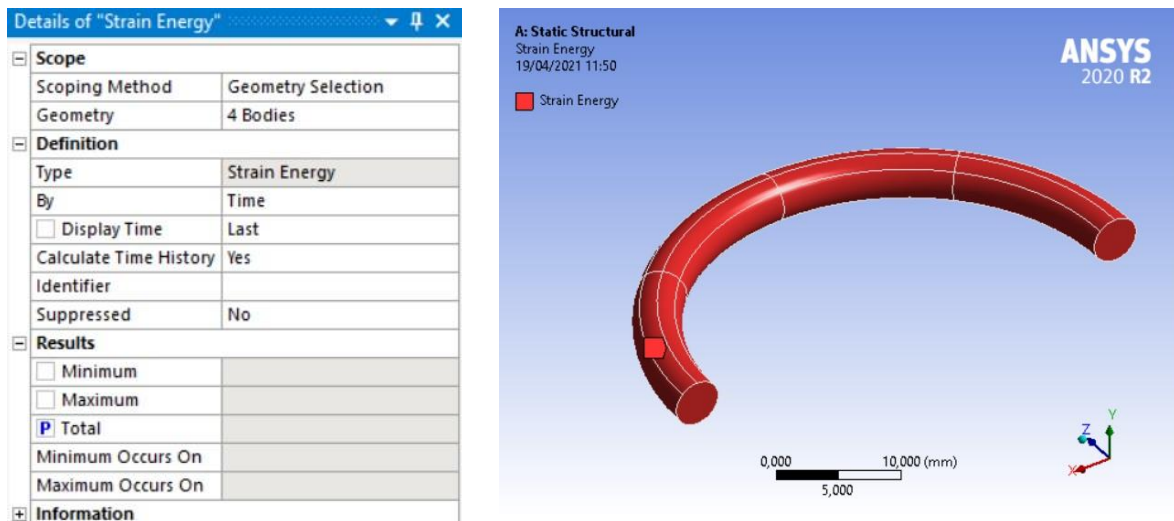
Figura 3.12: Energia di deformazione accumulata dalla semi-spira
