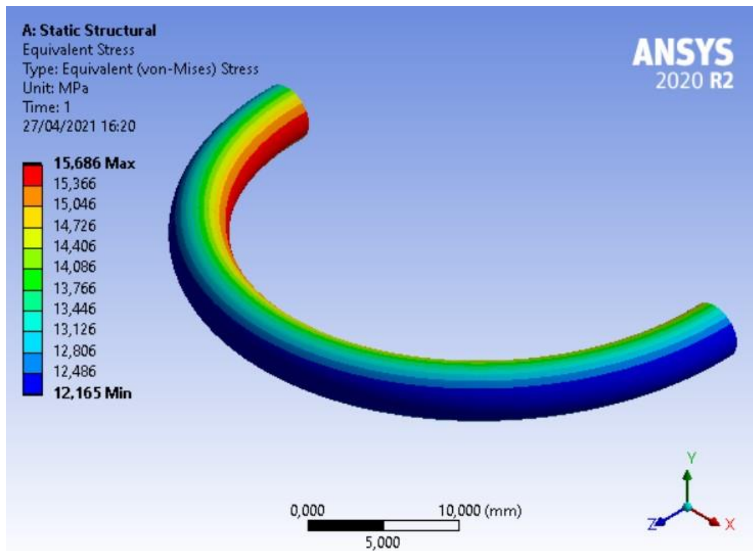
Figura 4.2: Tensioni di Von Mises sul mantello della semi-spira originaria
