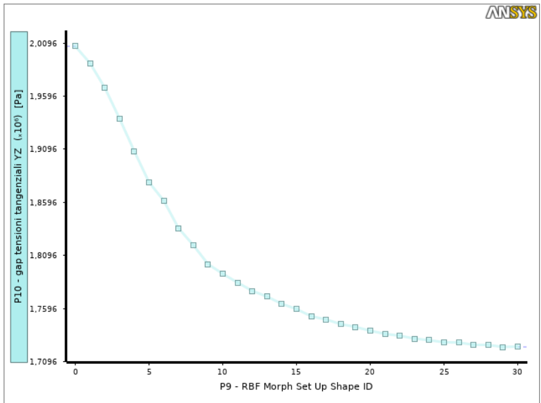
Figura 6: Gap degli sforzi tangenziali tra intradosso ed estradosso
