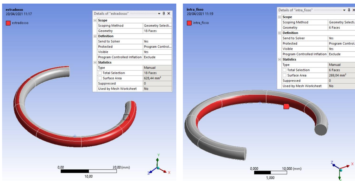
Figura 3.21: Creazione di estradosso ed intra_fisso
