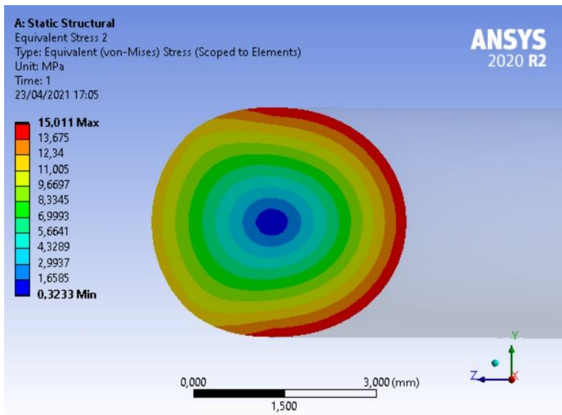
Figura 4.5: Tensioni di Von Mises sulla generica sezione della semi-spira finale
