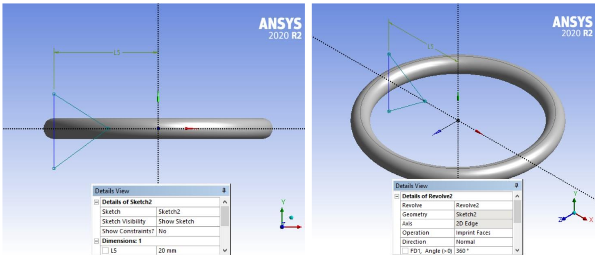
Figura 3.4: Secondo step di modellazione
