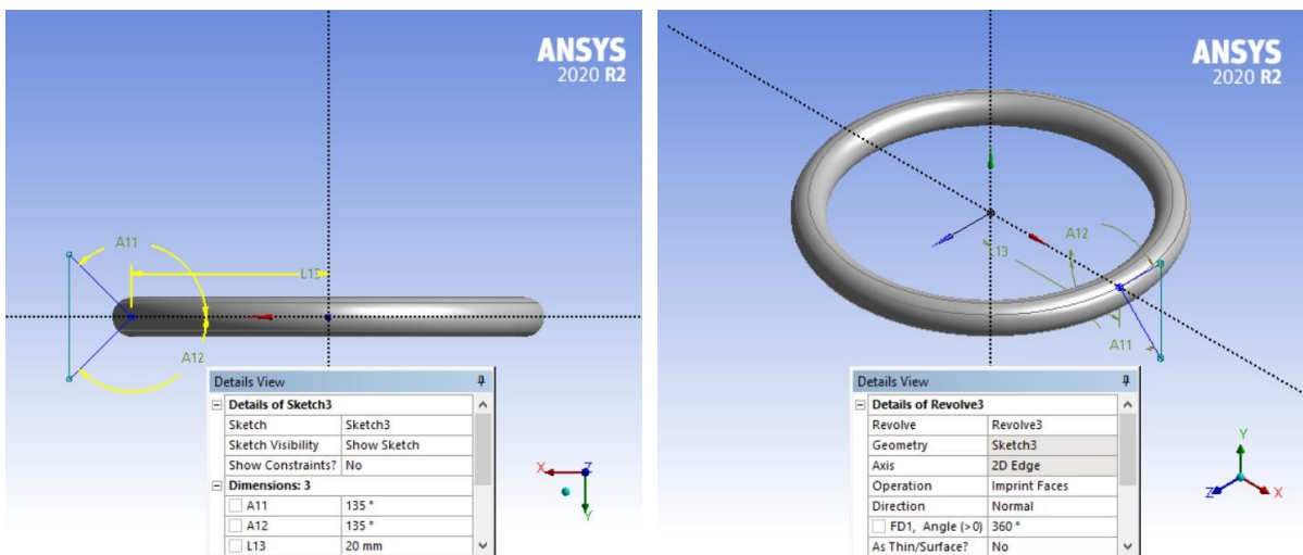
Figura 3.5: Terzo step di modellazione
