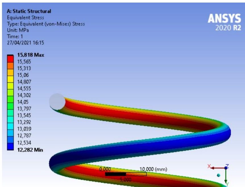
Figura 4.12: Tensioni di Von Mises sul mantello dell'elica originaria
