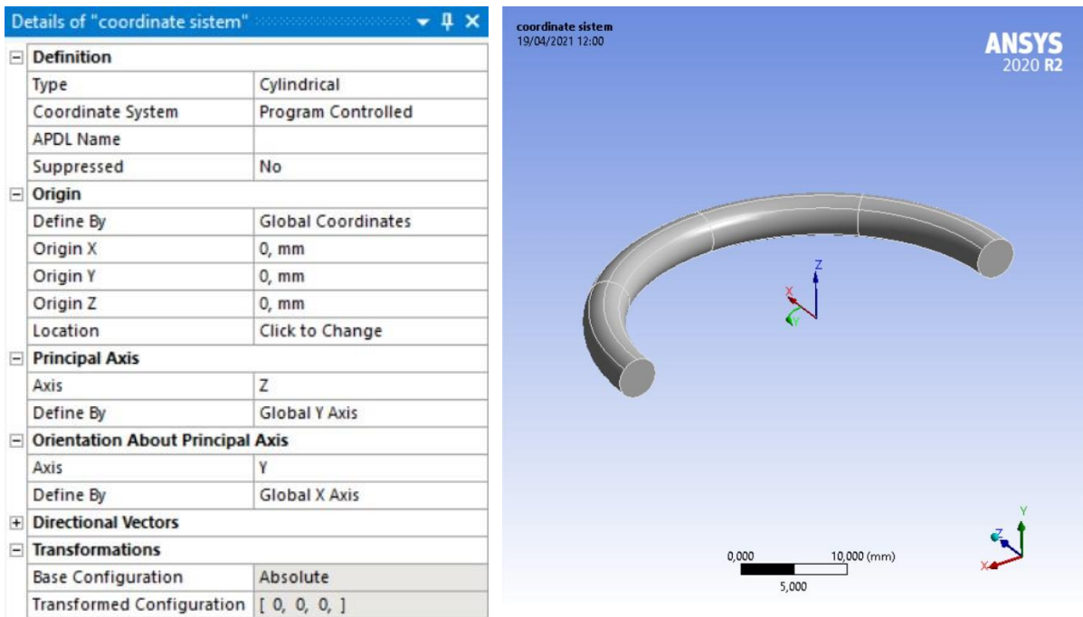
Figura 3.15: Riferimento a coordinate cilindriche "coordinate sistem"
