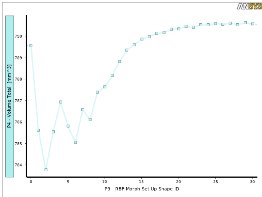
Figura 9: Volume totale della semi-spira
