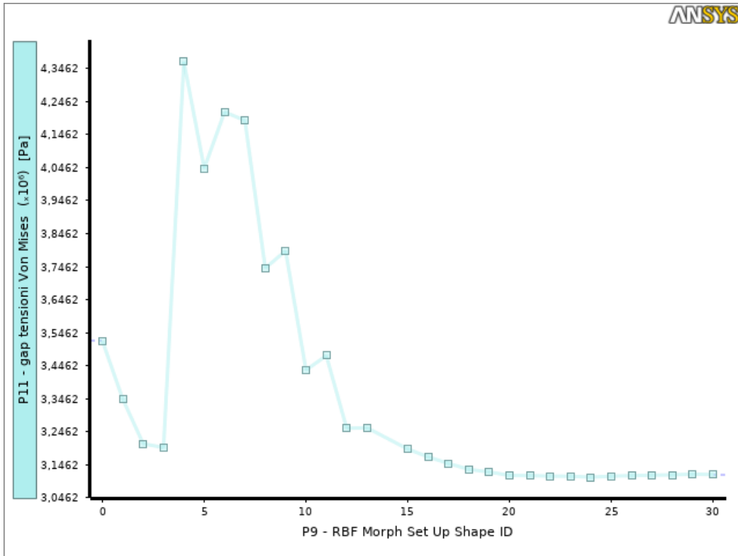
Figura 11: Gap tra massima e minima tensione di Von Mises
