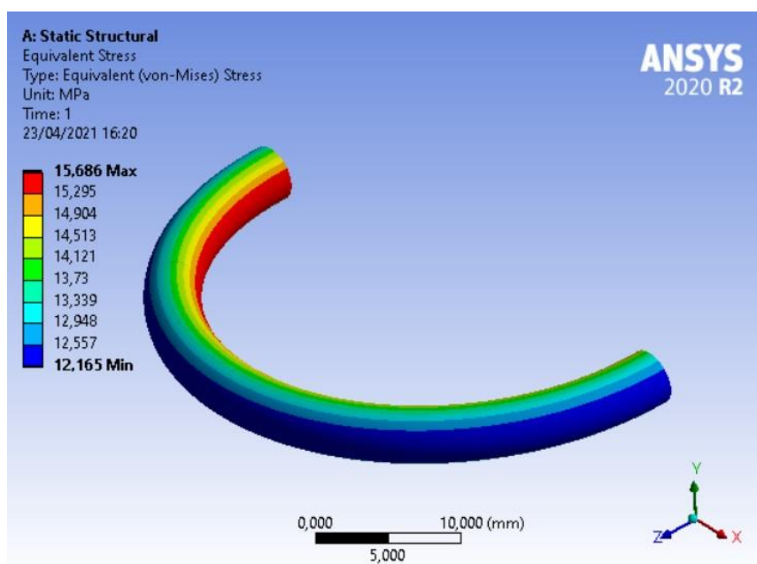
Figura 1.1: Campo degli sforzi sul mantello di una semi-spira piana della molla elicoidale (valutato in termini di tensione equivalente secondo il criterio di Von Mises)
