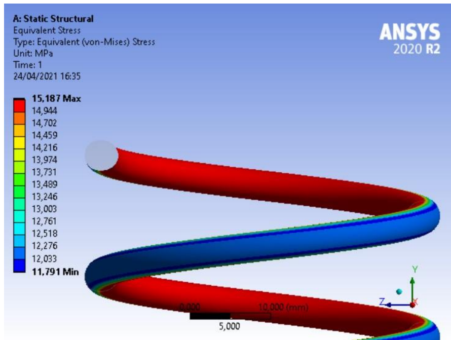
Figura 4.13: Tensioni di Von Mises sul mantello dell'elica ottimizzata
