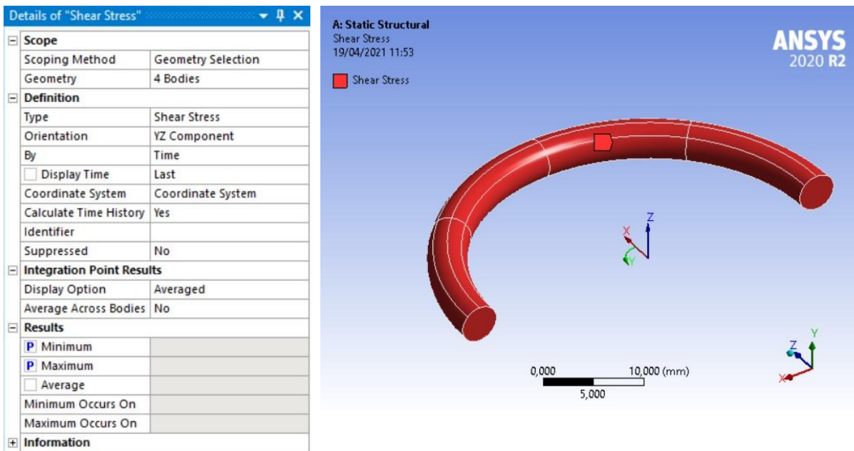
Figura 3.14: Tensioni tangenziali \tau_{zy} valutate nel sistema di riferimento "coordinate sistem"
