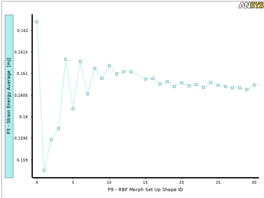
Figura 15: Energia di deformazione
