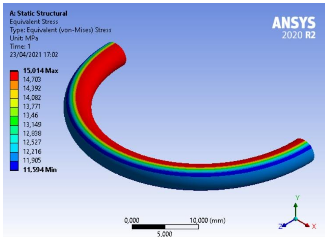
Figura 4.3: Tensioni di Von Mises sul mantello della semi-spira finale
