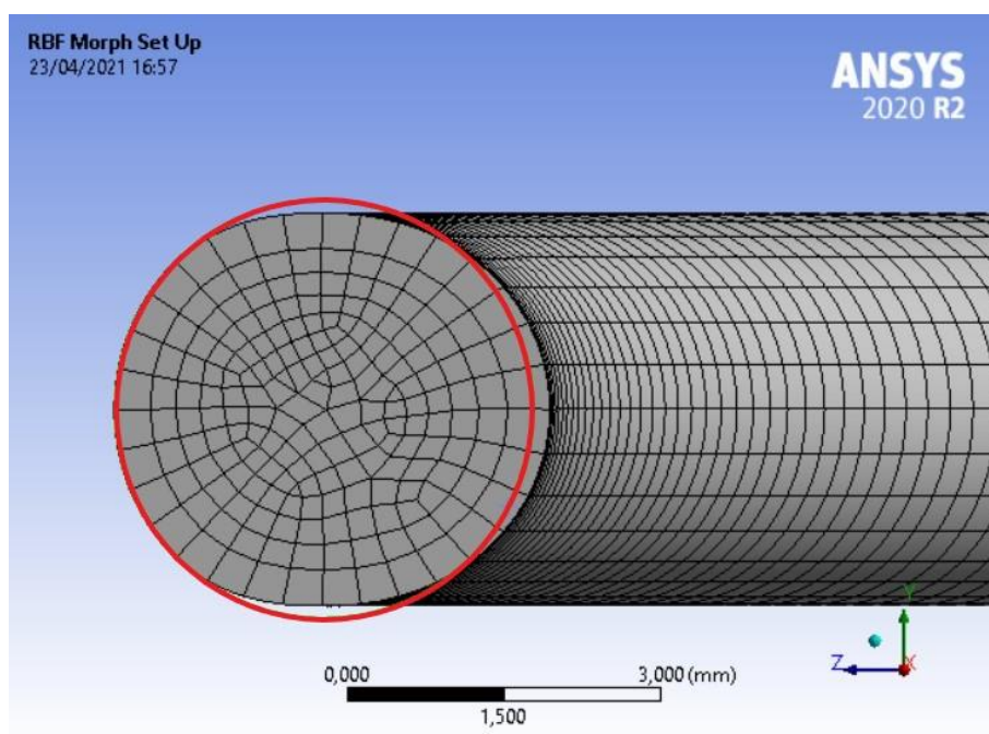
Figura 4.1: Sezione della semi-spira finale confrontata a quella originaria
