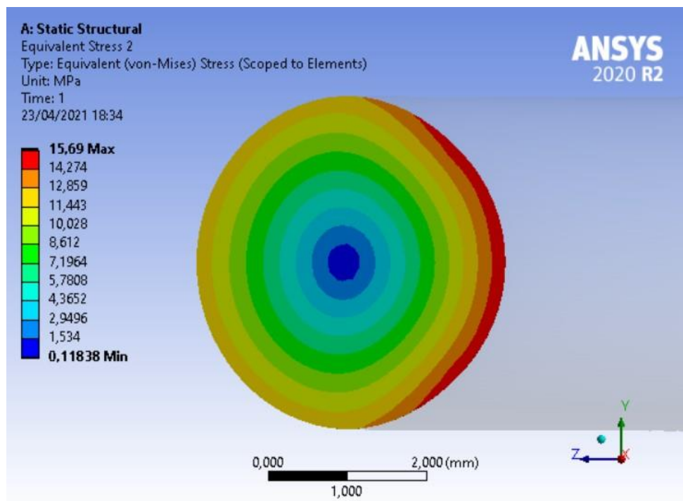
Figura 4.8: Tensioni di Von Mises sulla generica sezione della semi-spira finale
