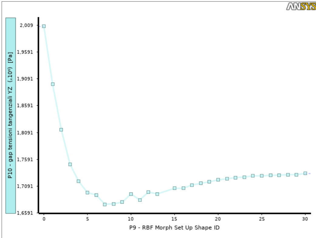
Figura 13: Gap tra gli sforzi tangenziali all'intradosso e all'estradosso
