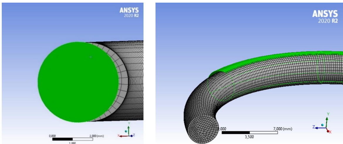
Figura 2: forma della semi-spira dopo 5 iterazioni del morphing
