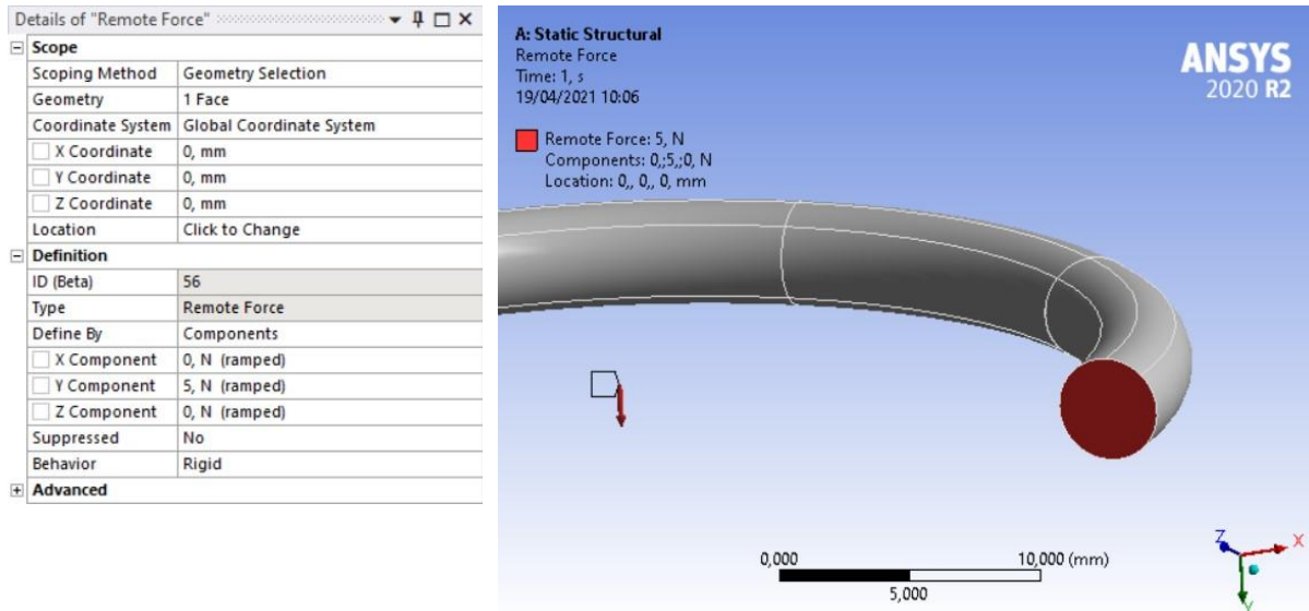
Figura 3.9: Settaggio dell'oggetto Remote Force
