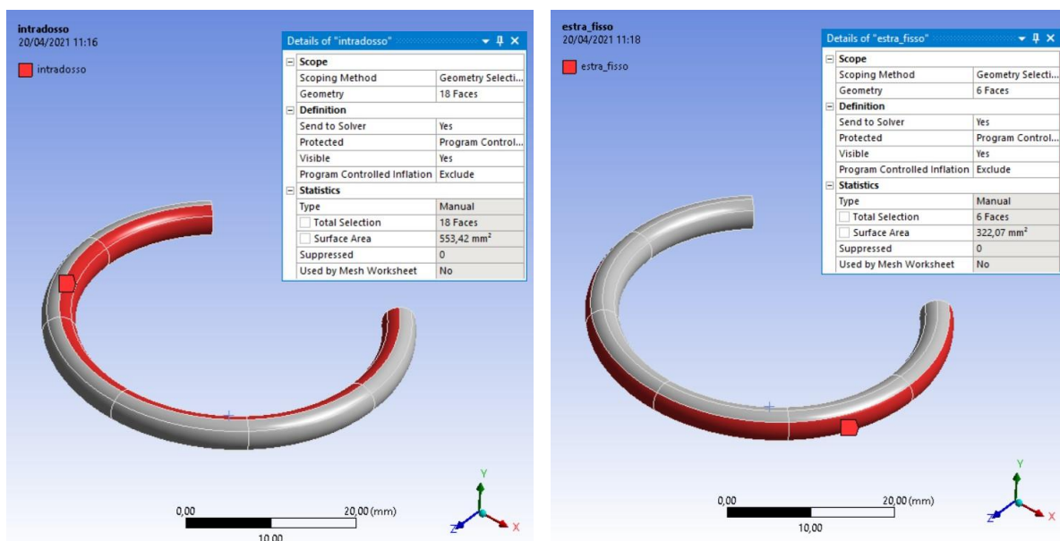
Figura 3.20: Creazione di intradosso ed estra_fisso
