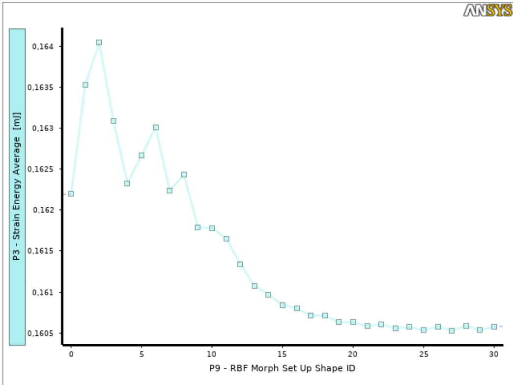
Figura 7: Energia di deformazione
