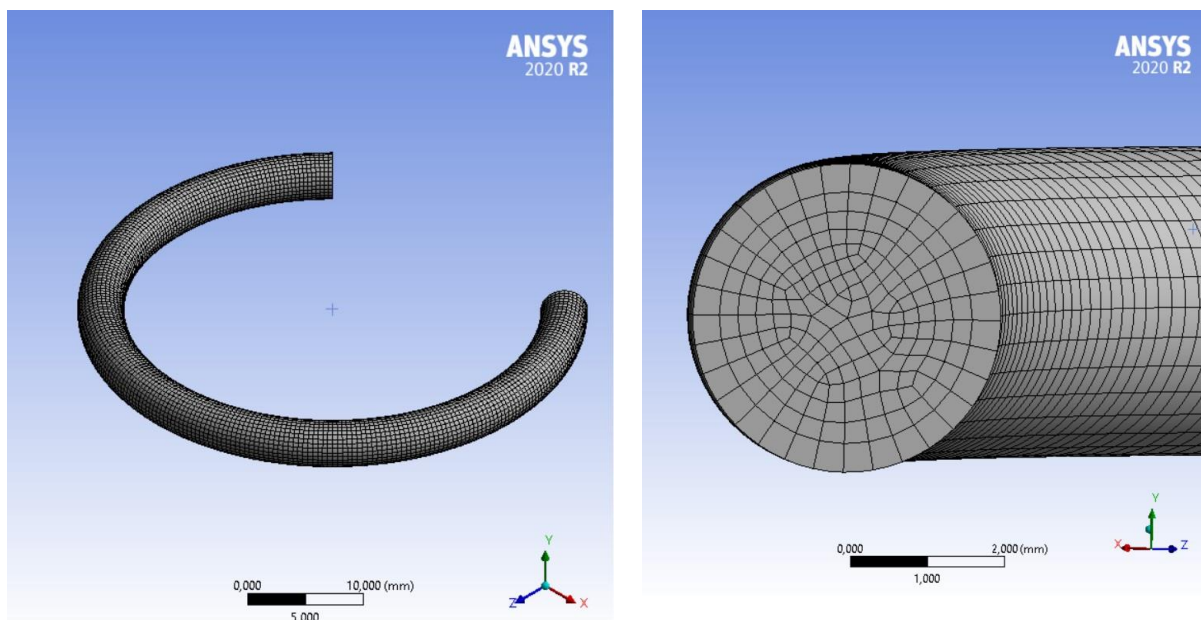
Figura 3.18: Discretizzazione del modello
