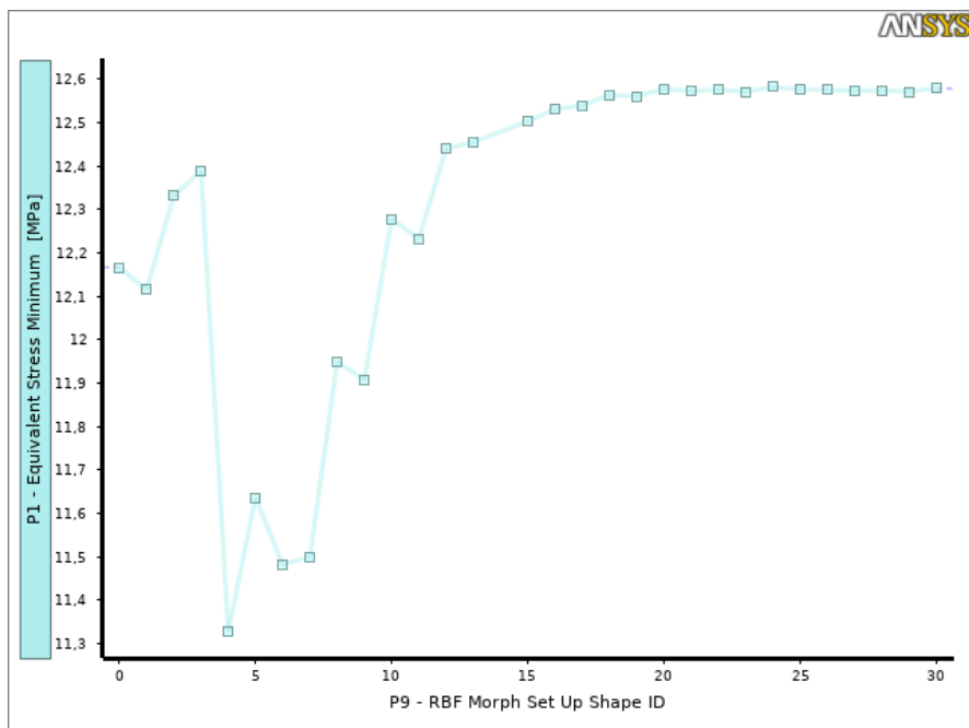
Figura 10: Minima tensione di Von Mises
