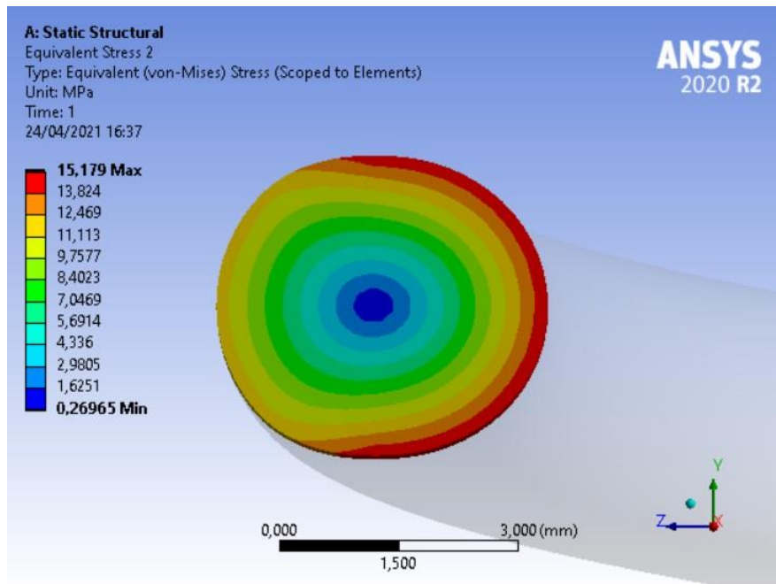
Figura 4.11: Tensioni di Von Mises sulla generica sezione del filo d'elica ottimizzato
