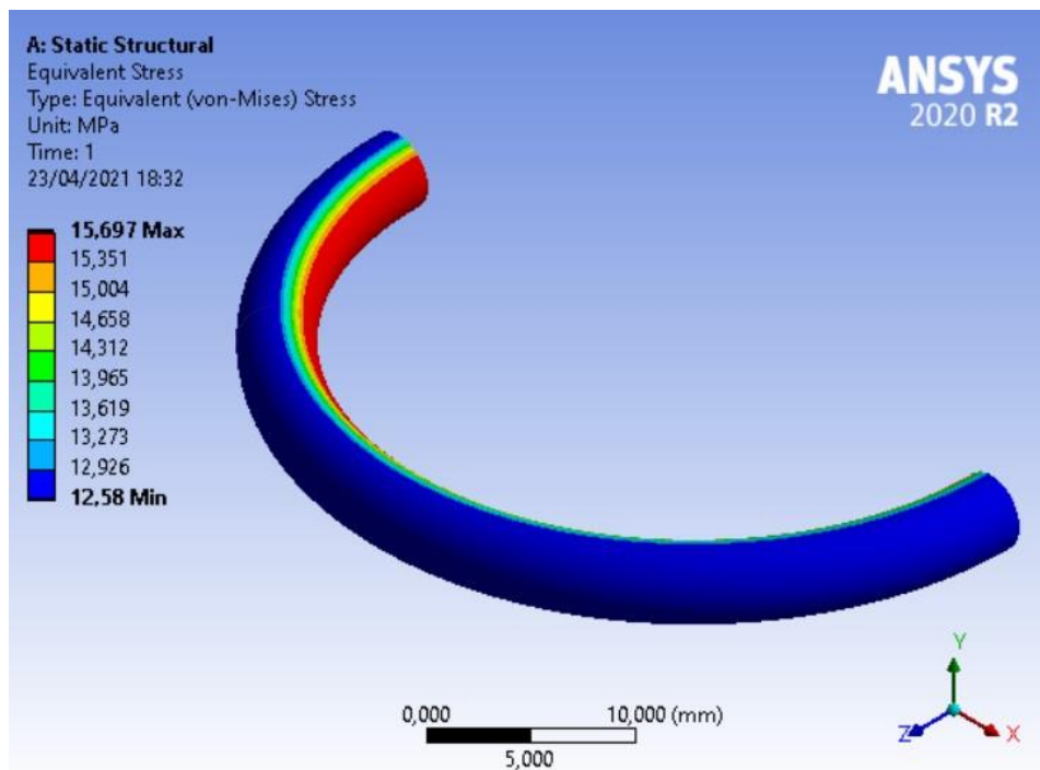
Figura 4.7: Tensioni di Von Mises sul mantello della semi-spira finale
