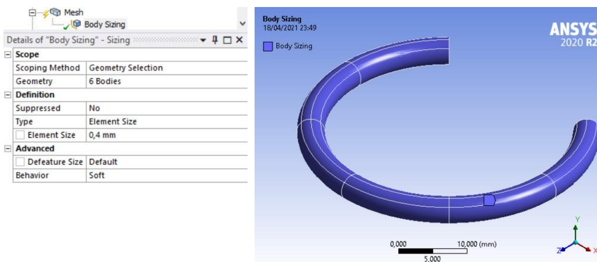
Figura 3.19: Impostazione del Body Sizing
