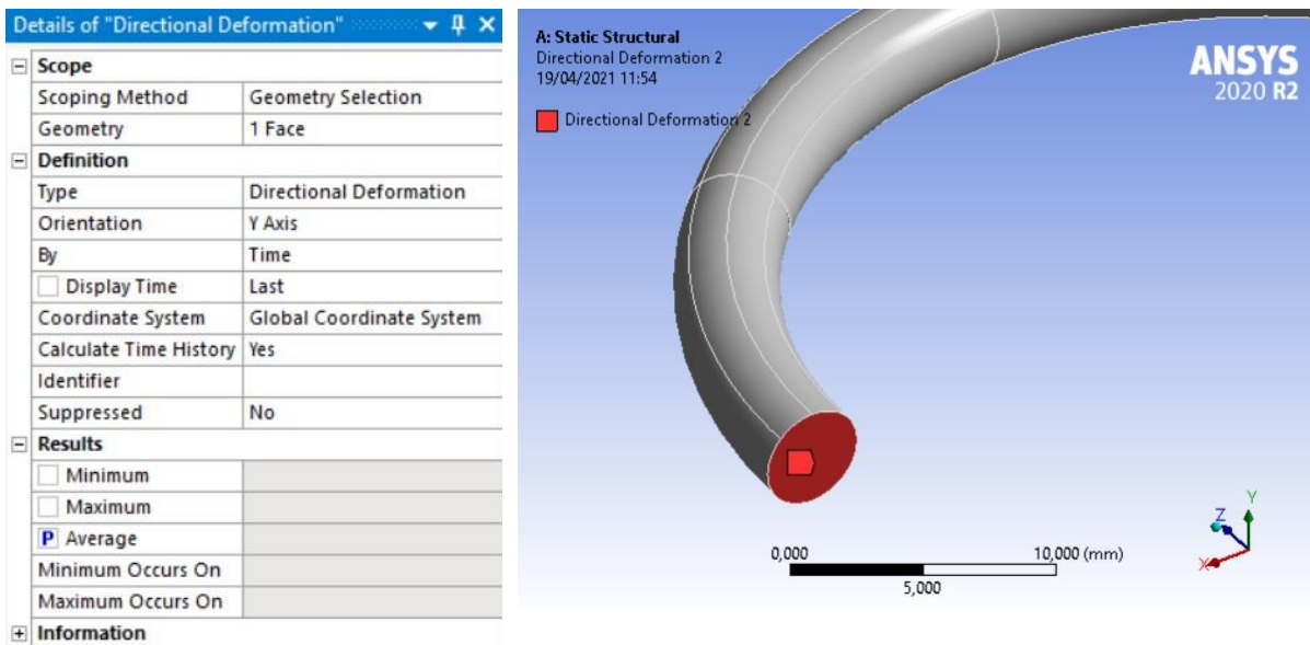
Figura 3.16: Abbassamento della sezione parallelo all'asse della semi-spira
