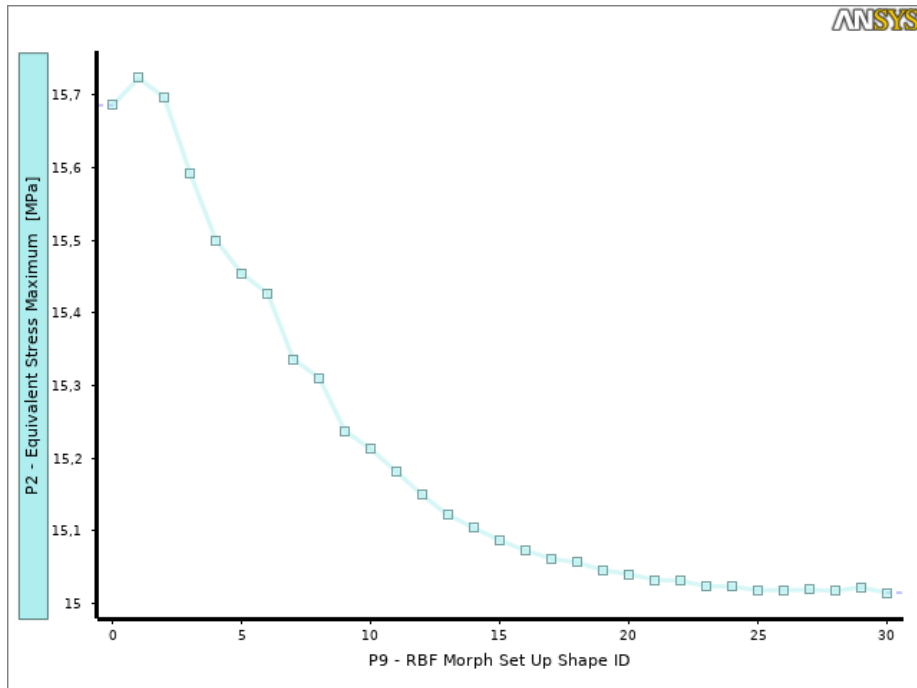
Figura 3: Massima tensione di Von Mises
